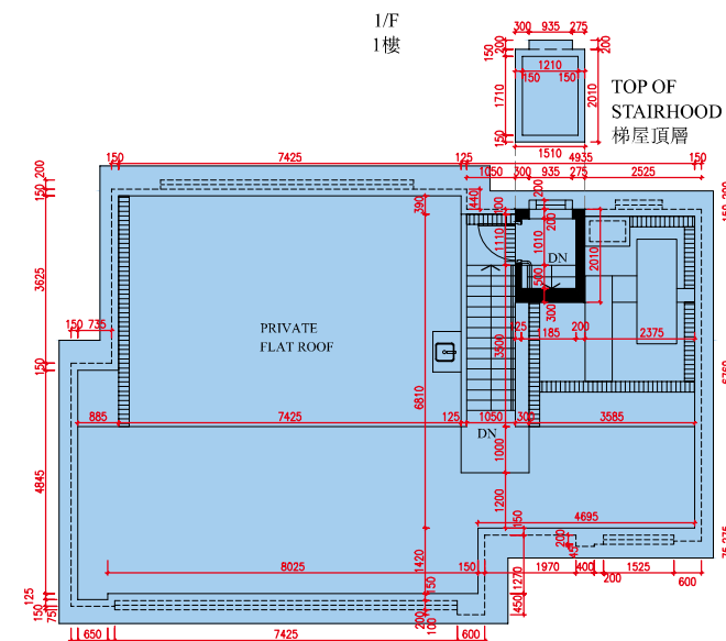
R/F 天台
