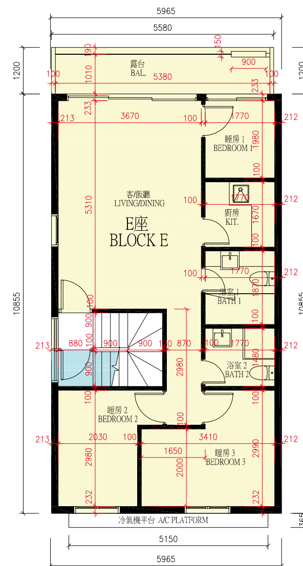
First Floor Plan 一樓樓面平面圖
