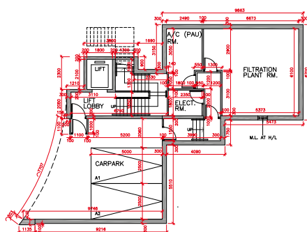
CARPARK LEVEL PLAN 停車場層平面圖
