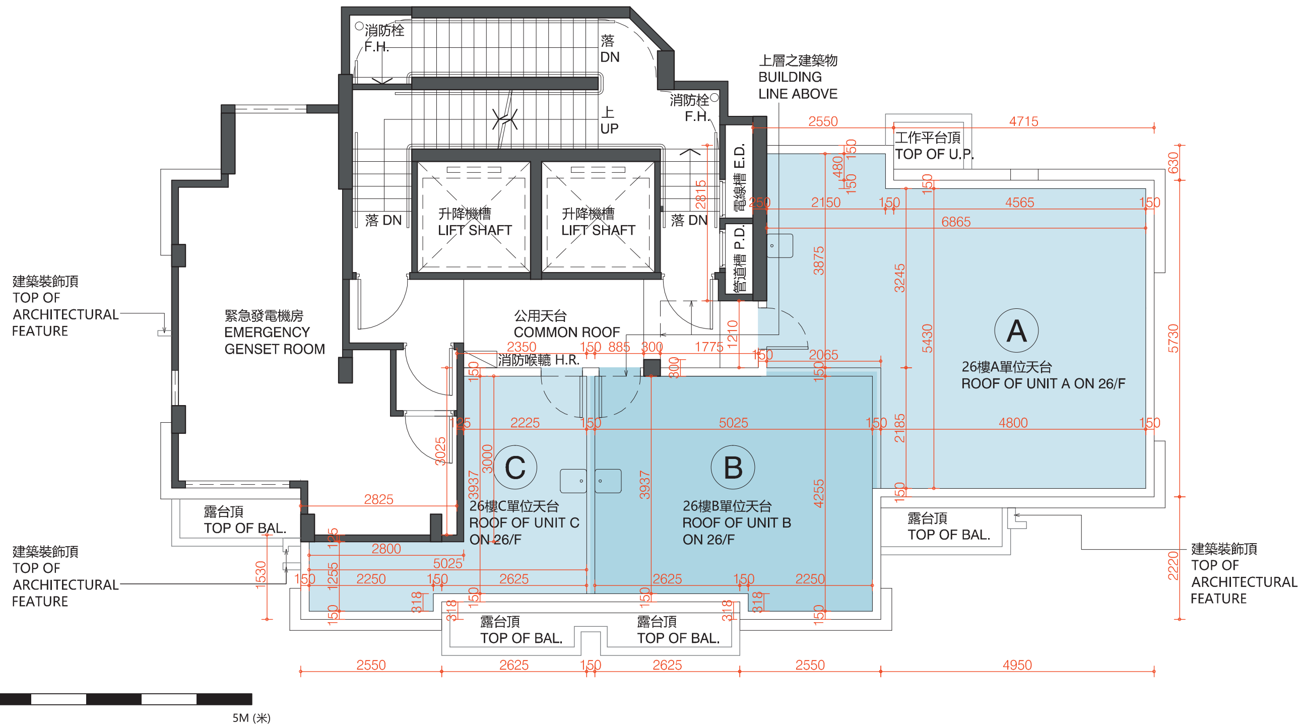
Roof Floor Plan 天台樓面平面圖
