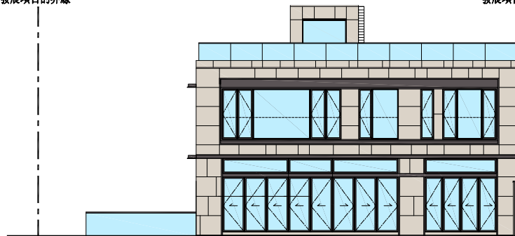
ELEVATION C 立面圖 C
