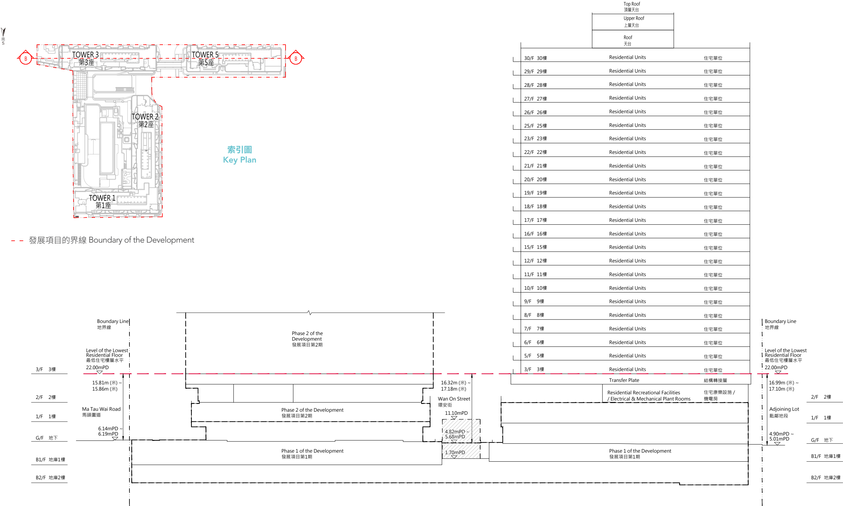
橫截面圖 B-B Cross-Section Plan B-B
