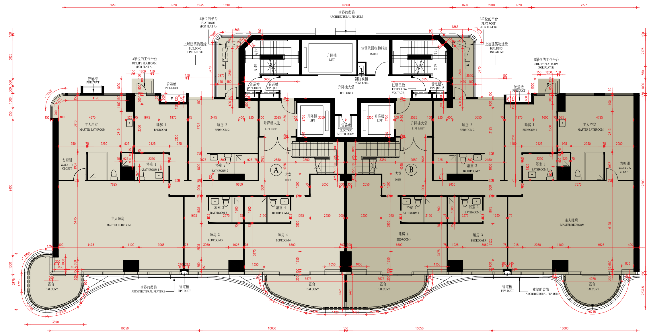
TOWER 1 17/F FLOOR PLAN 第1座 17樓平面圖
