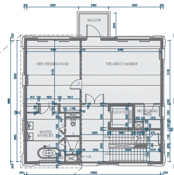
Floor Plan 2/F 二樓平面圖
