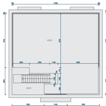
Floor Plan R/F 天台平面圖
