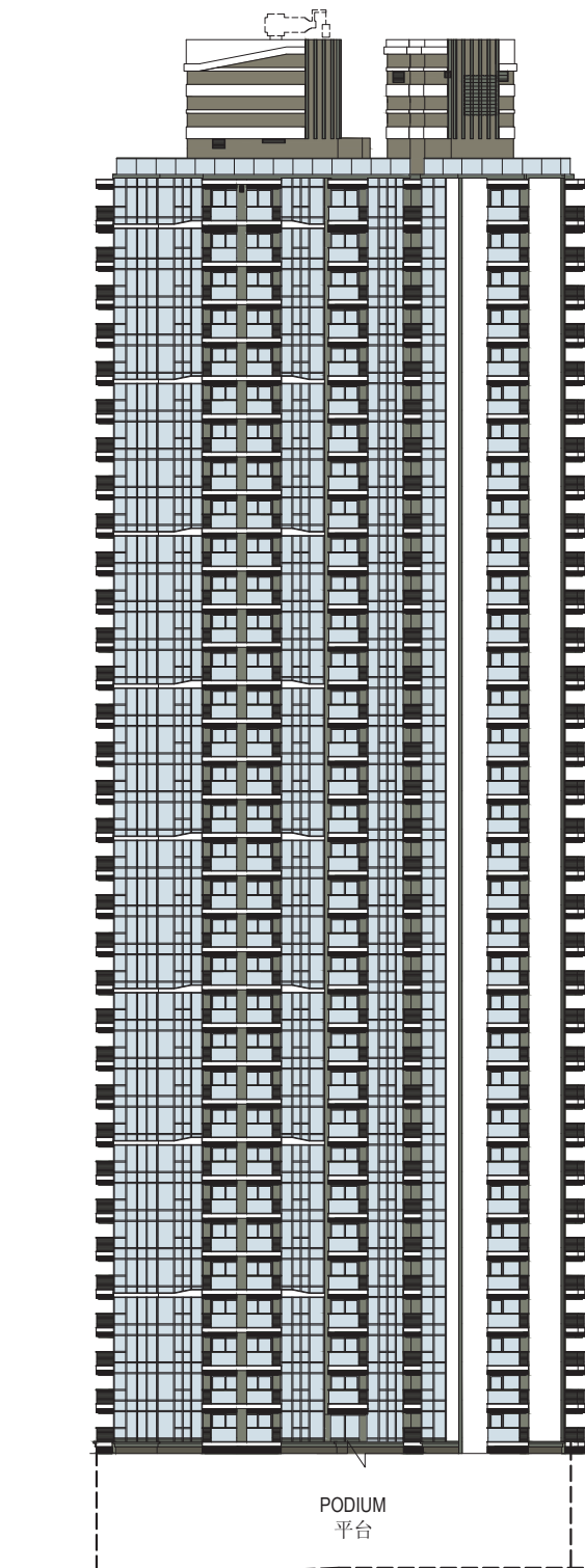
ELEVATION PLAN 4 立面圖 4
