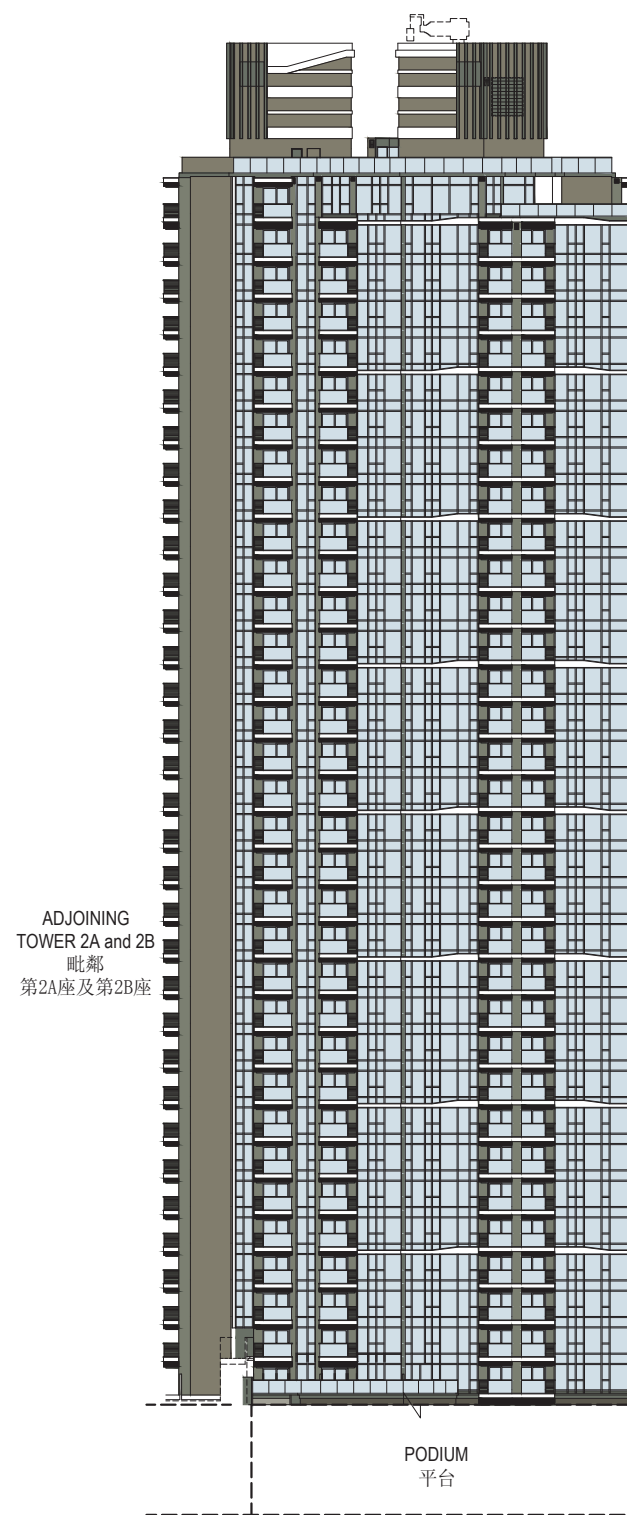
ELEVATION PLAN 2 立面圖 2
