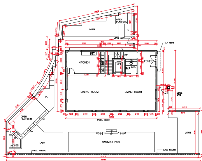
GROUND FLOOR PLAN 地下平面圖
