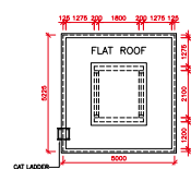
TOP ROOF PLAN 頂層天台平面圖
