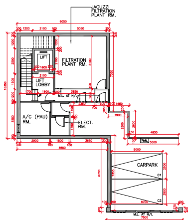
CARPARK LEVEL PLAN 停車場層平面圖
