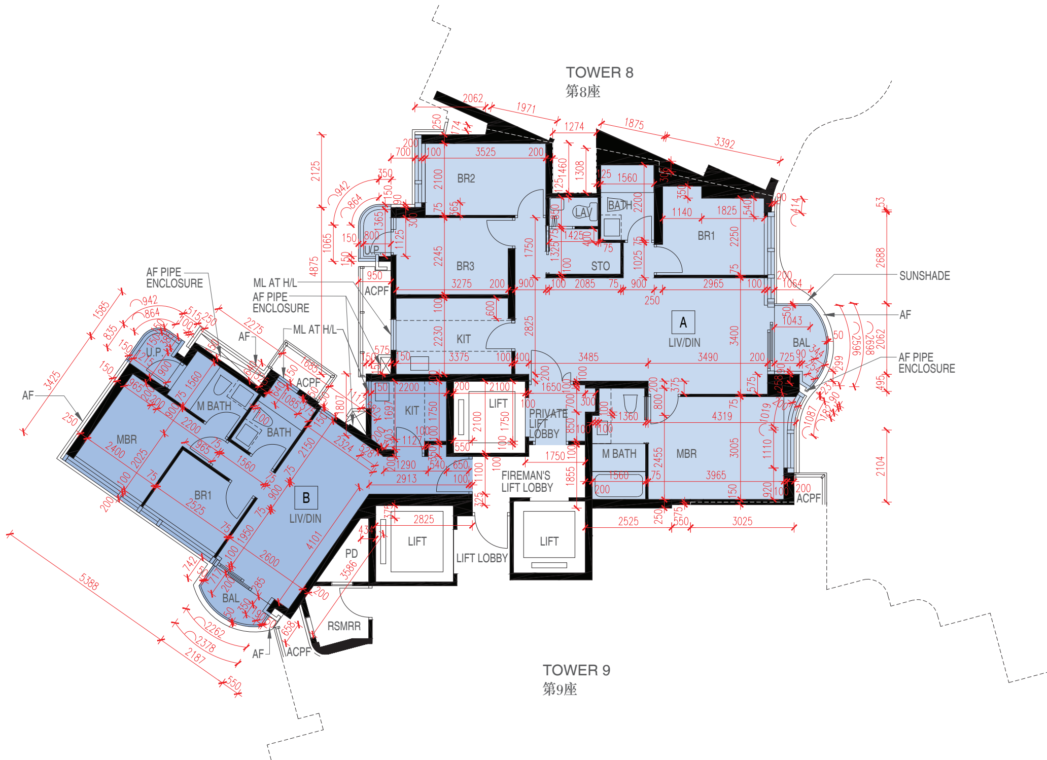
TOWER 9A 26/F 第9A座 26樓
