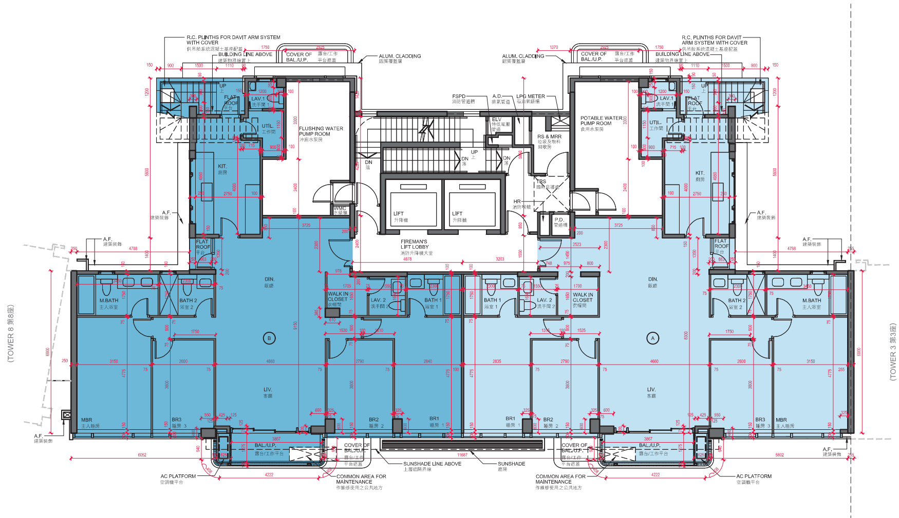
TOWER 6 16/F FLOOR PLAN 第6座 16樓樓面平面圖
