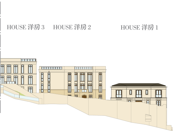
Elevation 4 立面圖四
