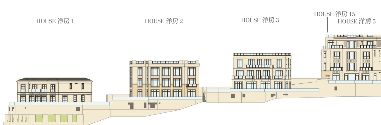
Elevation 1 立面圖一
