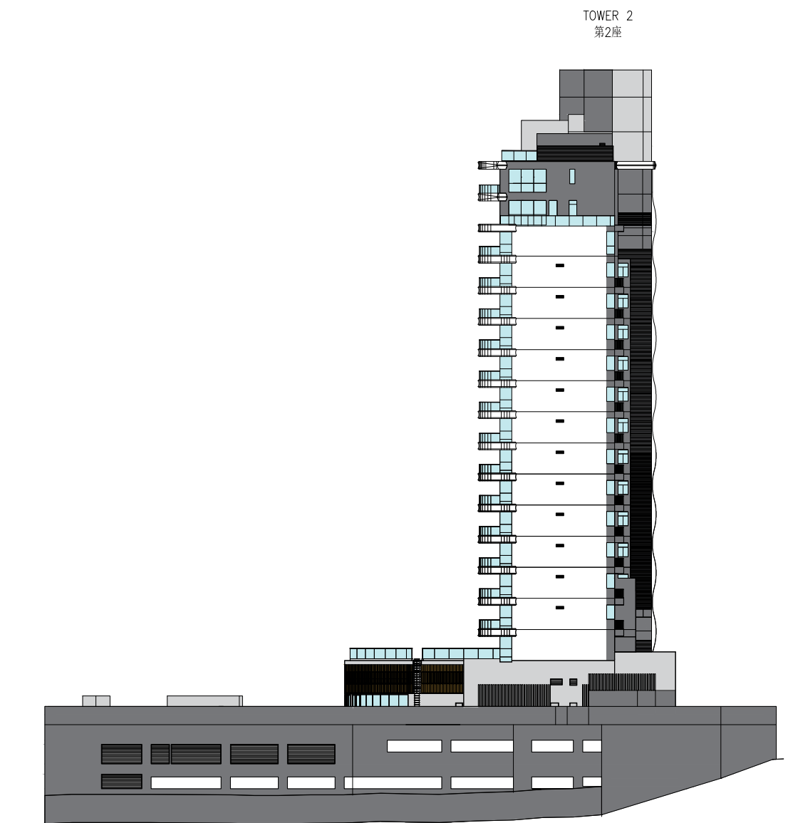
ELEVATION 2 立面 2
