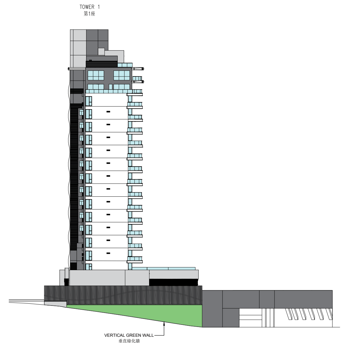
ELEVATION 4 立面 4
