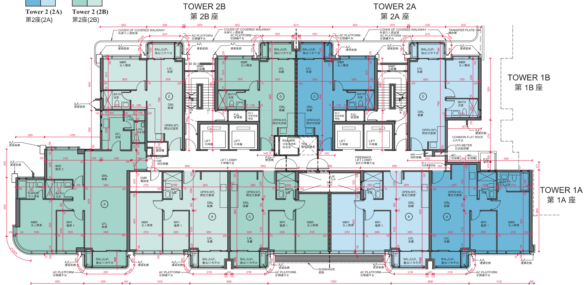
TOWER 2A & 2B 2/F FLOOR PLAN 第2A座及第2B座 2樓樓面平面圖
