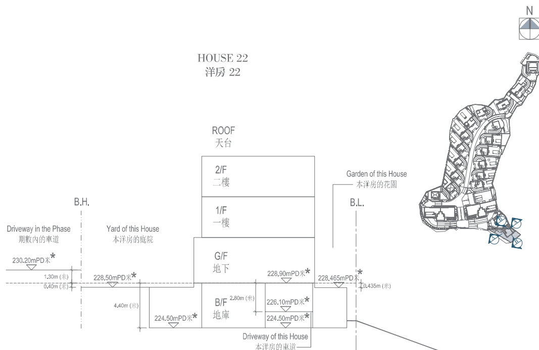
Section A 剖面圖 A
