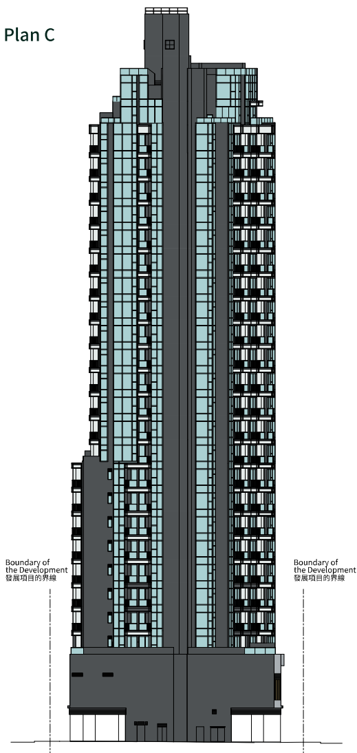
Elevation Plan D 立面圖 D
