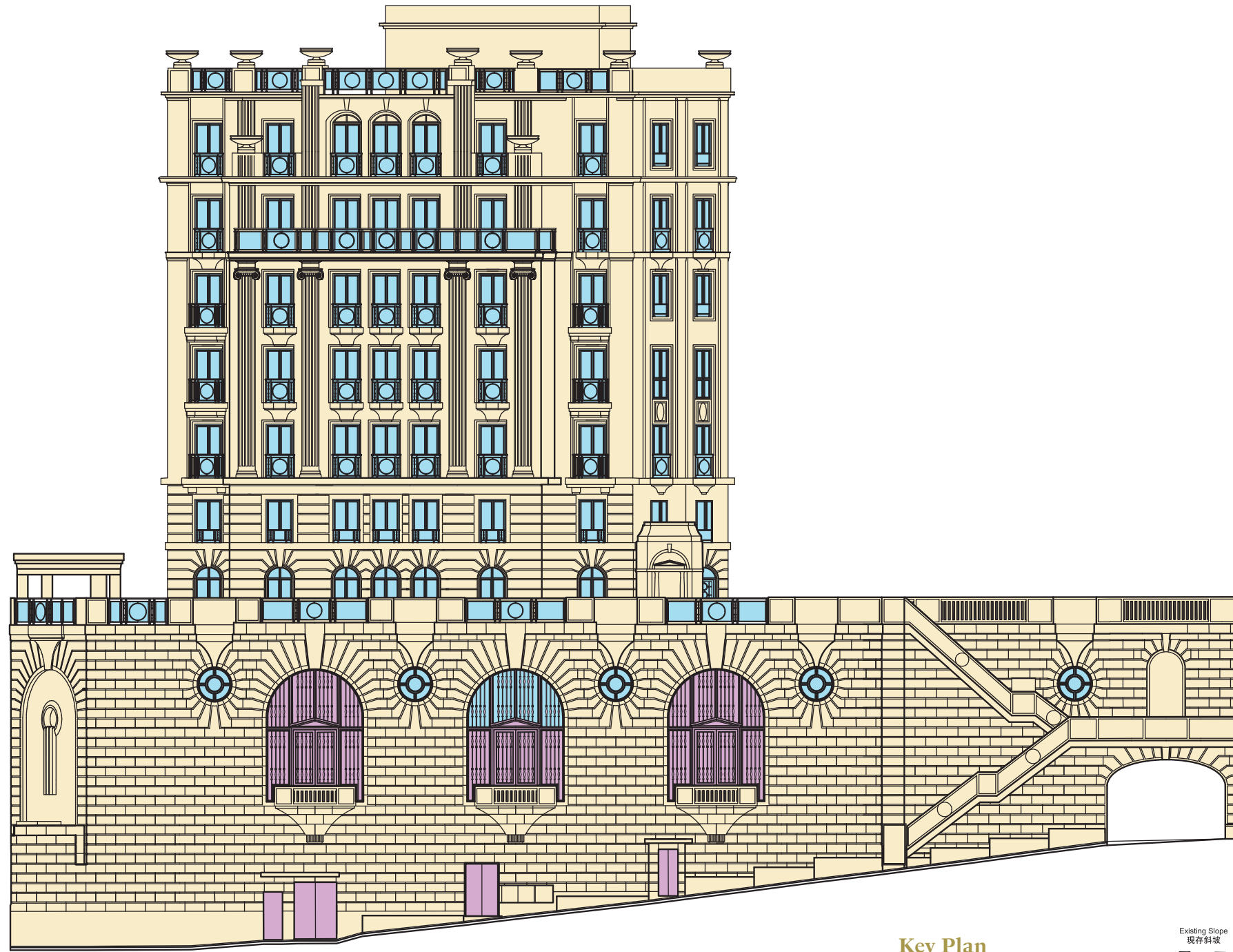
Front Elevation Plan 正面立面圖
