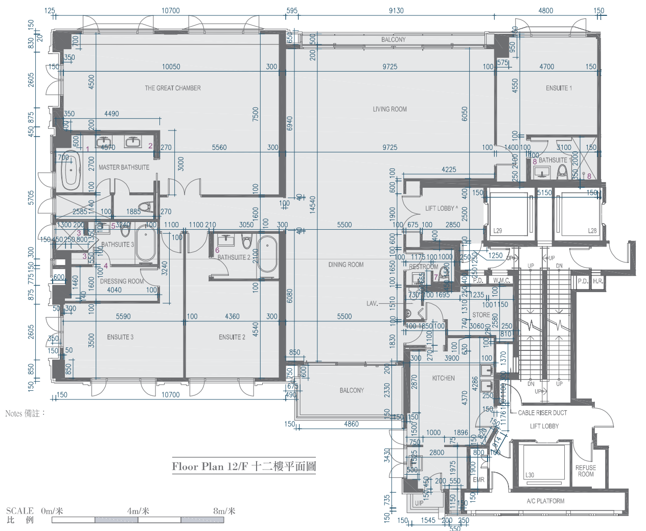
PLAN SHOWING LATEST LAYOUT* 現狀間隔平面圖*
