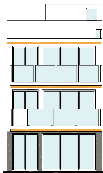
ELEVATION 1 立面圖一
