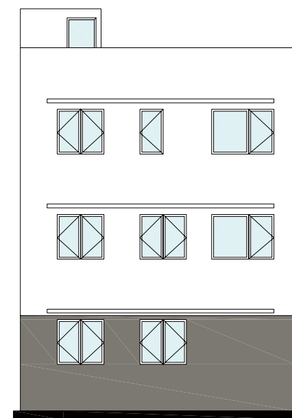
ELEVATION 3 立面圖三
