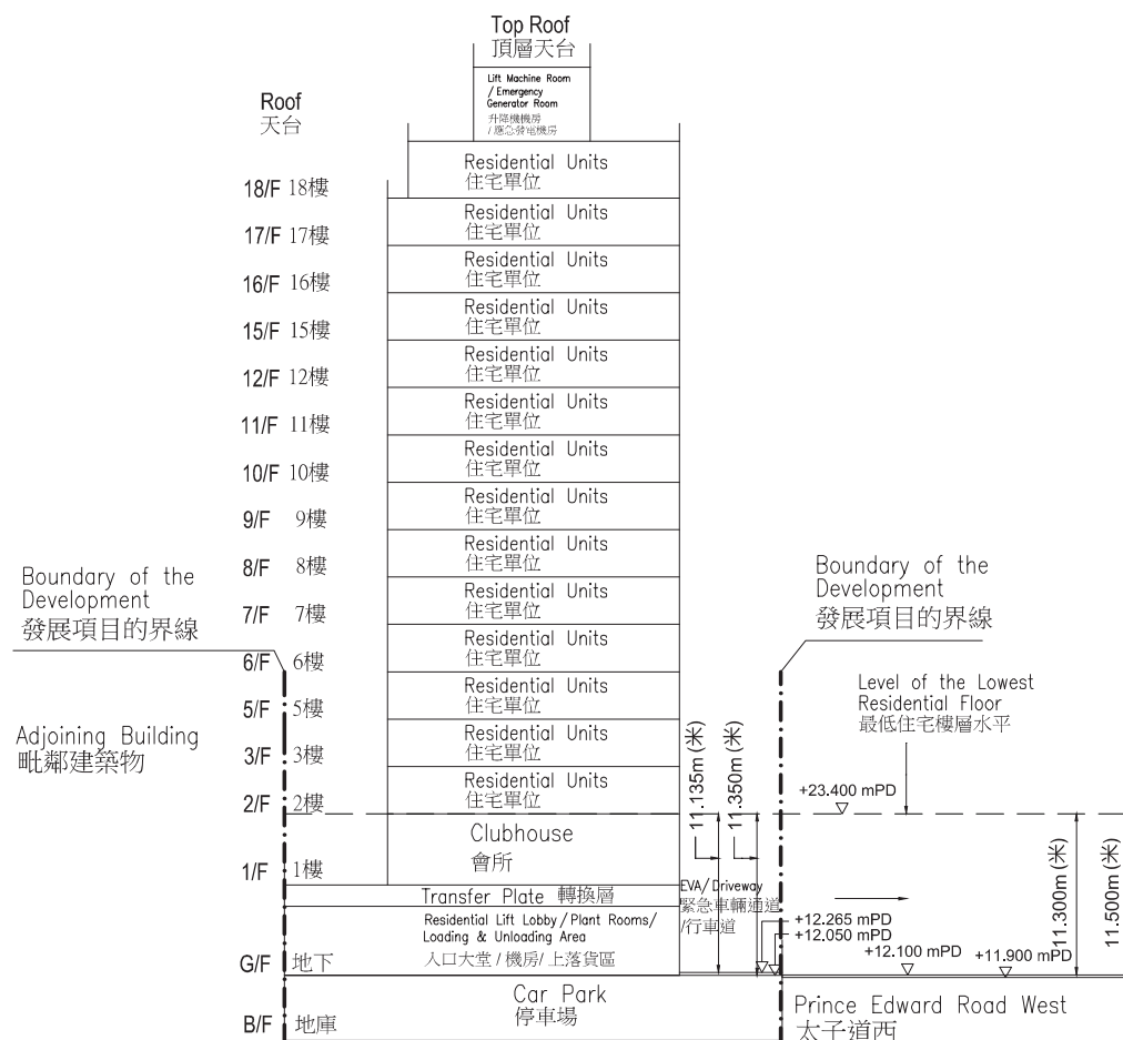
CROSS-SECTION PLAN A-A 橫截面圖 A-A
