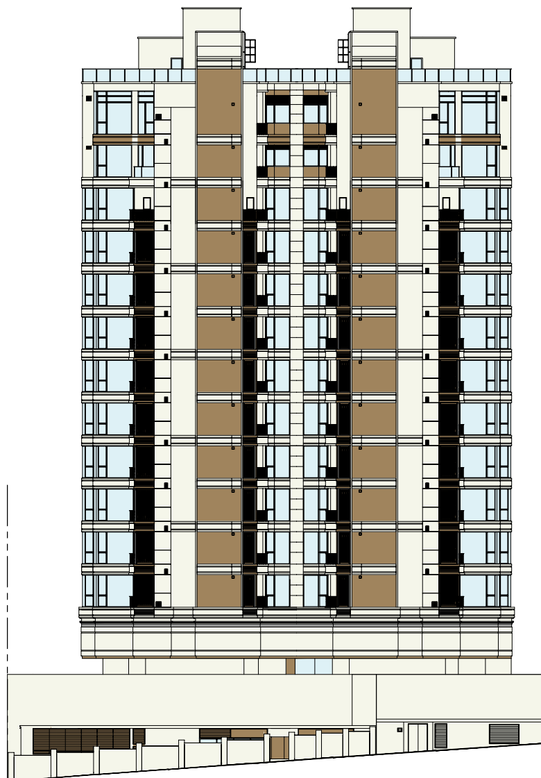
ELEVATION D 立面圖 D
