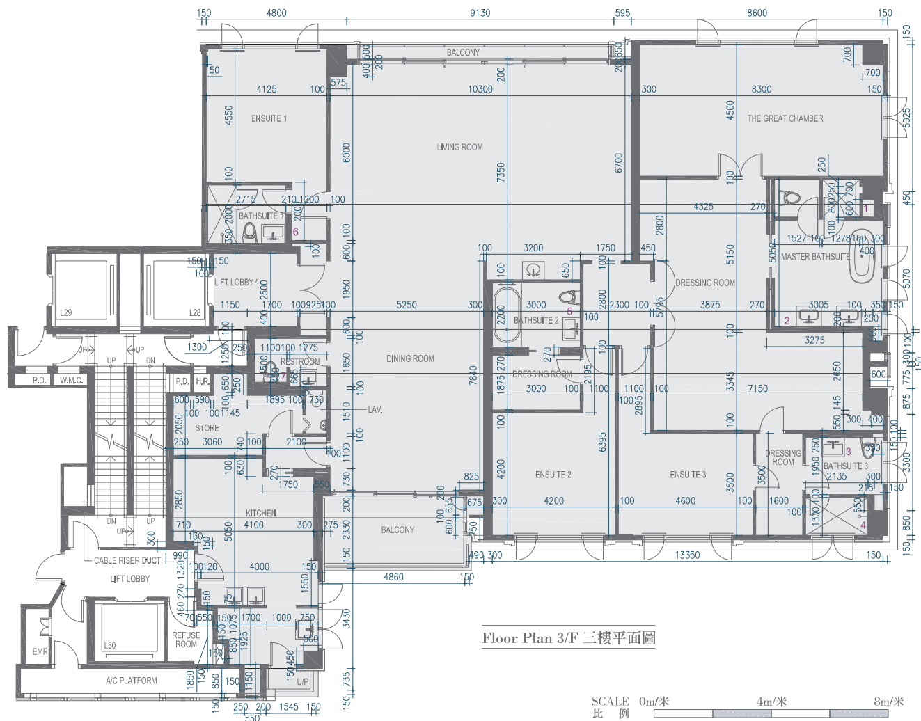
PLAN SHOWING LATEST LAYOUT* 現狀開隔平面圖*
