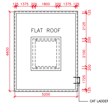
TOP ROOF PLAN 頂層天台平面圖
