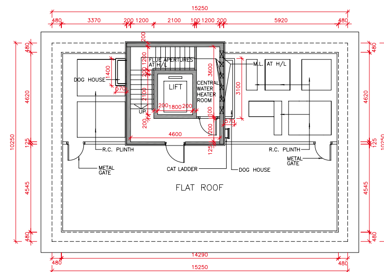
ROOF PLAN 天台平面圖
