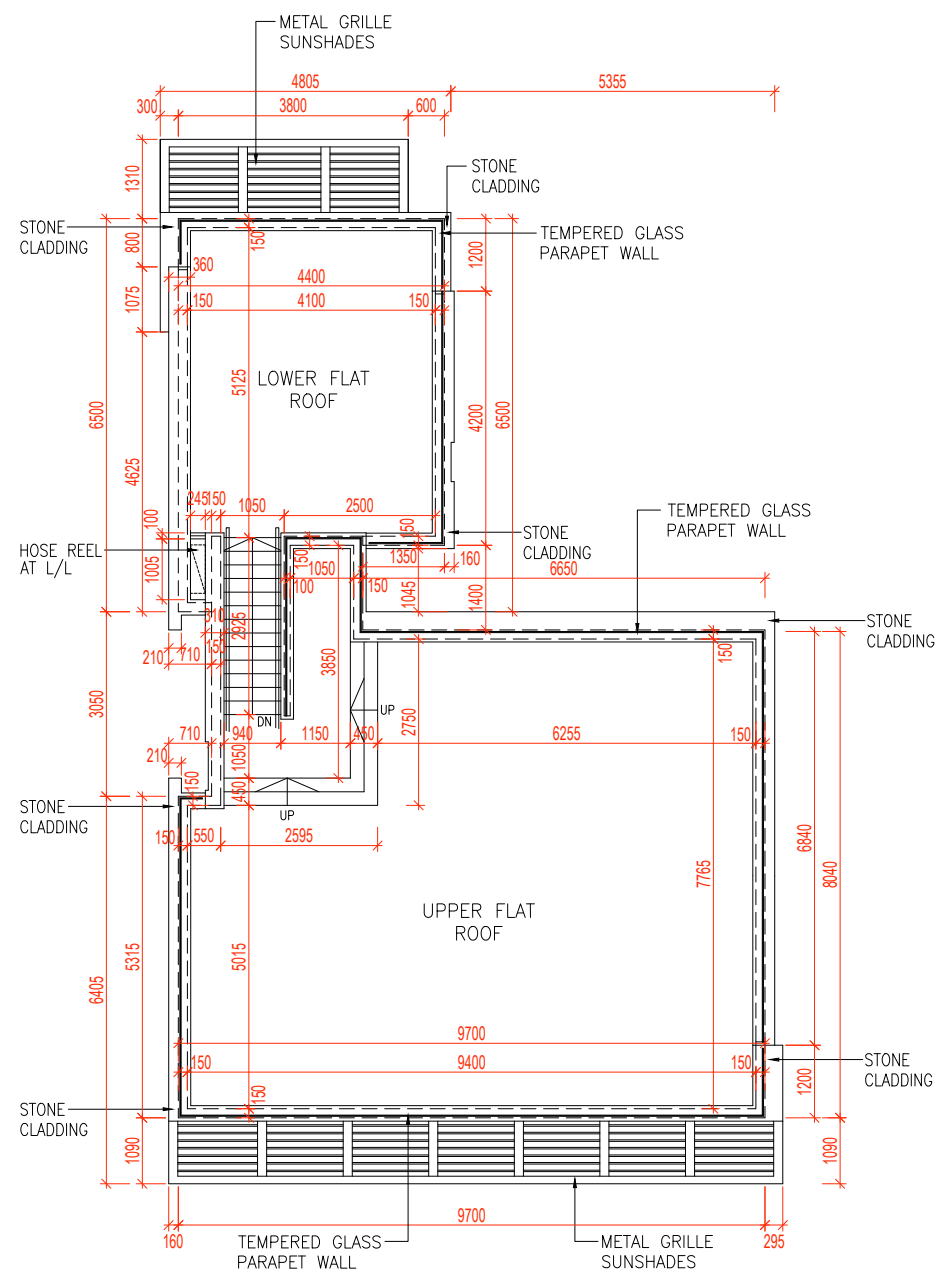
ROOF PLAN (R/F PLAN) 天台平面圖
