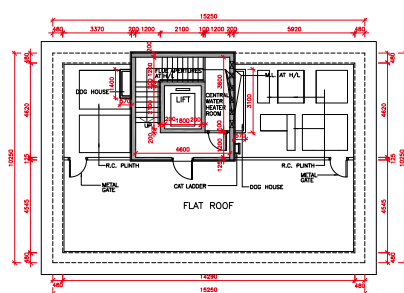
ROOF PLAN 天台平面圖
