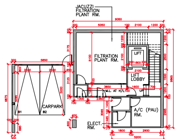
CARPARK LEVEL PLAN 停車場層平面圖
