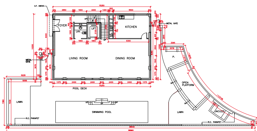
GROUND FLOOR PLAN 地下平面圖
