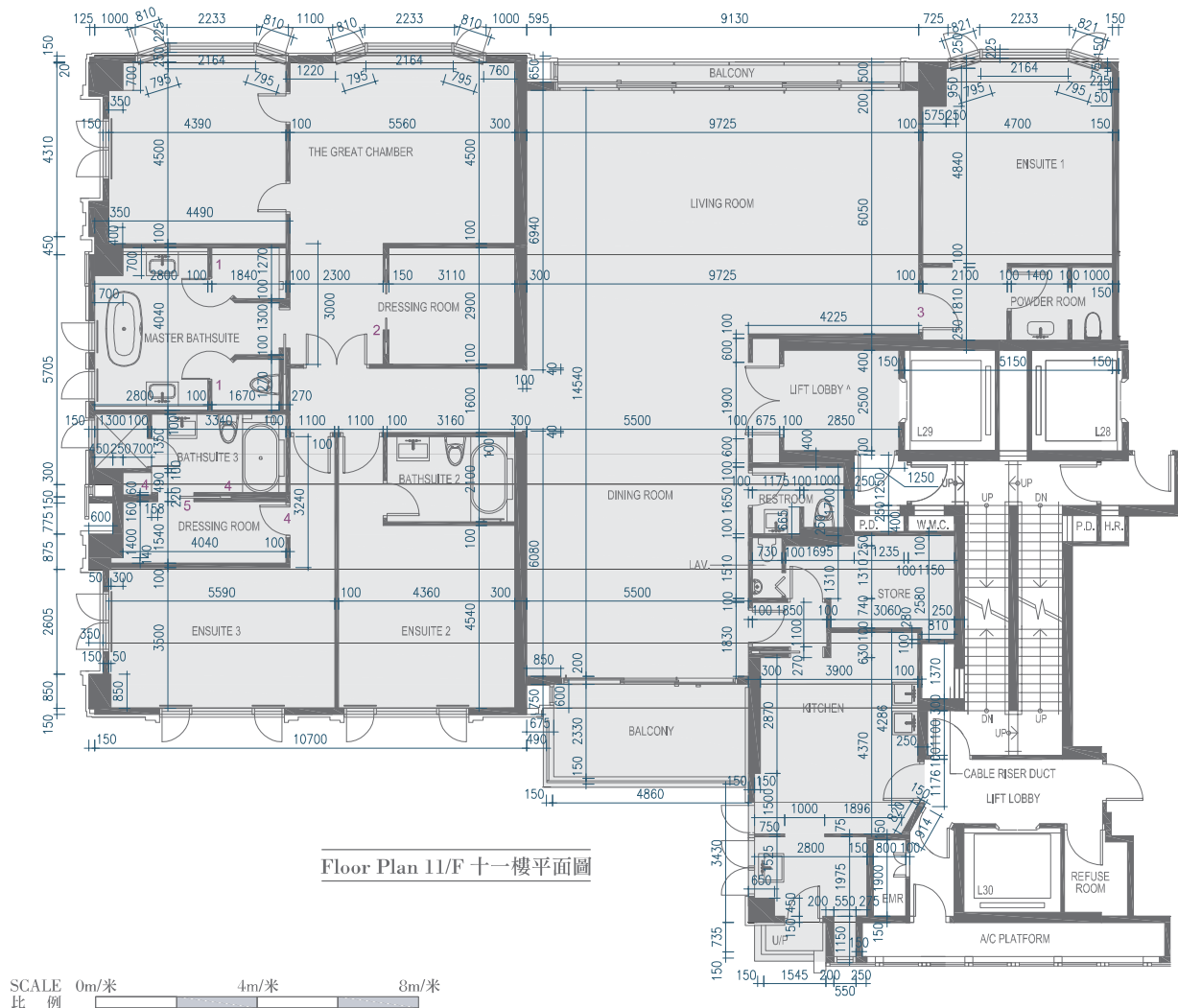
PLAN SHOWING LATEST LAYOUT* 現狀間隔平面圖*
