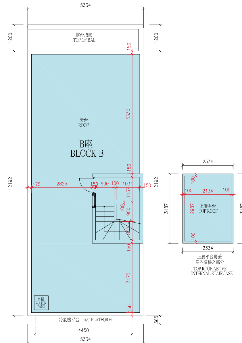
Roof Floor Plan 天台樓面平面圖
