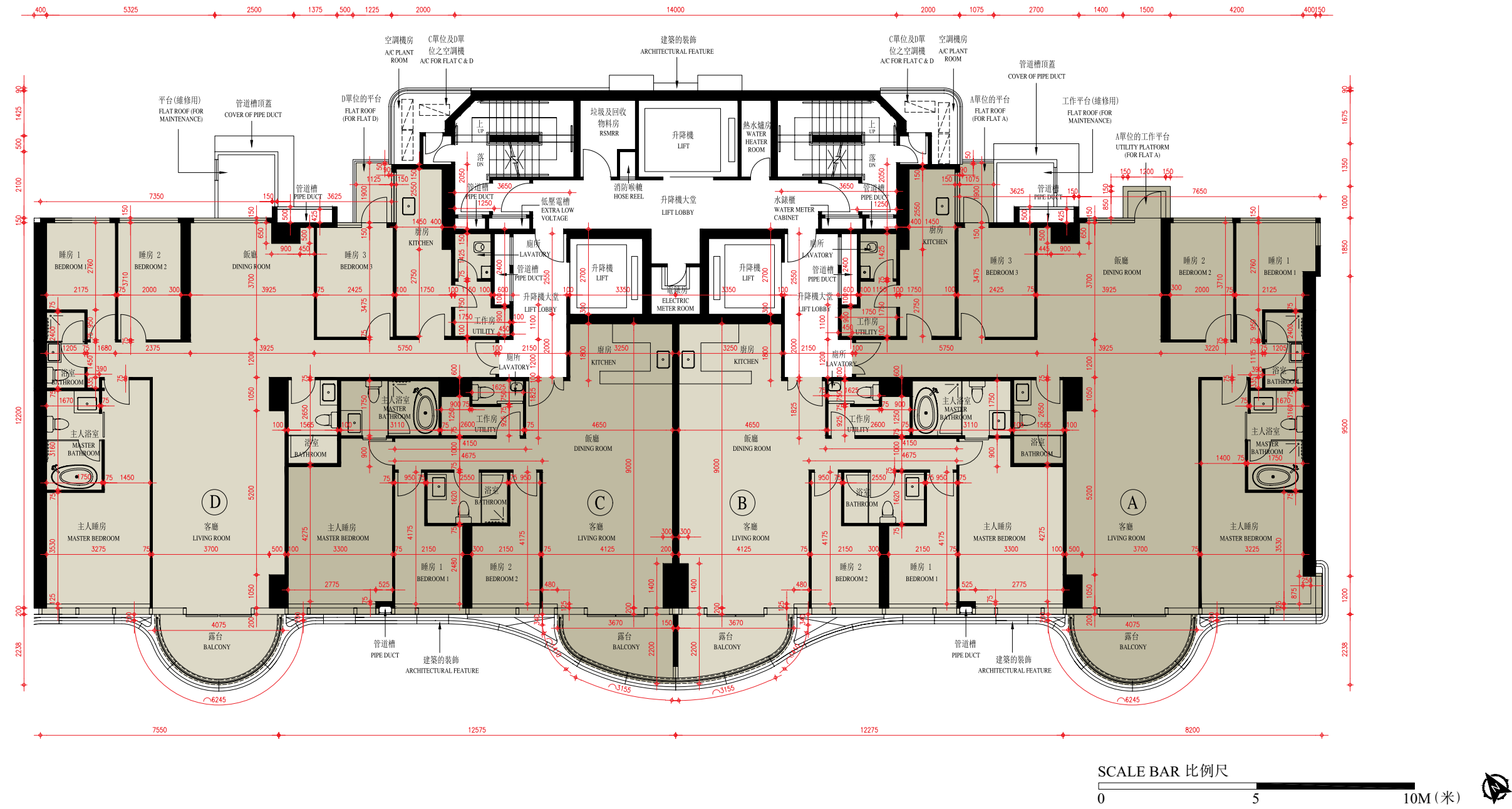
TOWER 2 3/F FLOOR PLAN 第2座3樓平面圖
