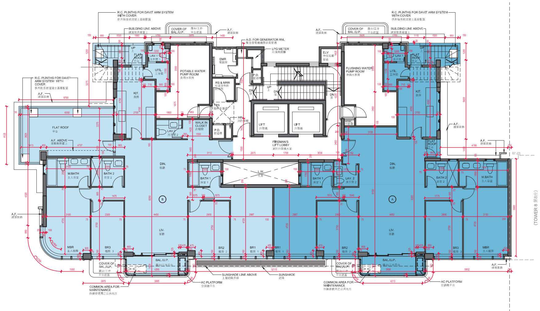
TOWER 9 16/F FLOOR PLAN 第9座 16樓樓面平面圖
