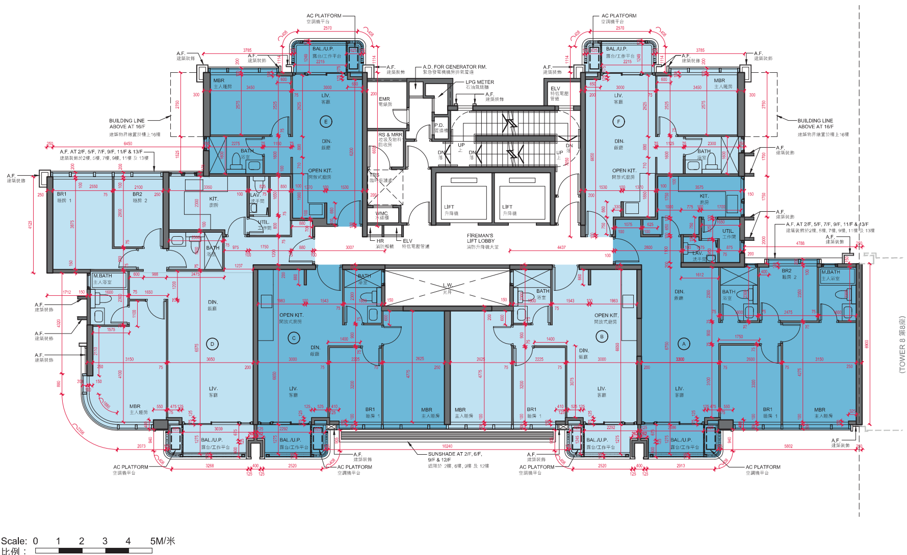
TOWER 9 2/F-3/F, 5/F-13/F, 15/F FLOOR PLAN 第9座 2樓至3樓，5樓至13樓，15樓樓面平面圖
