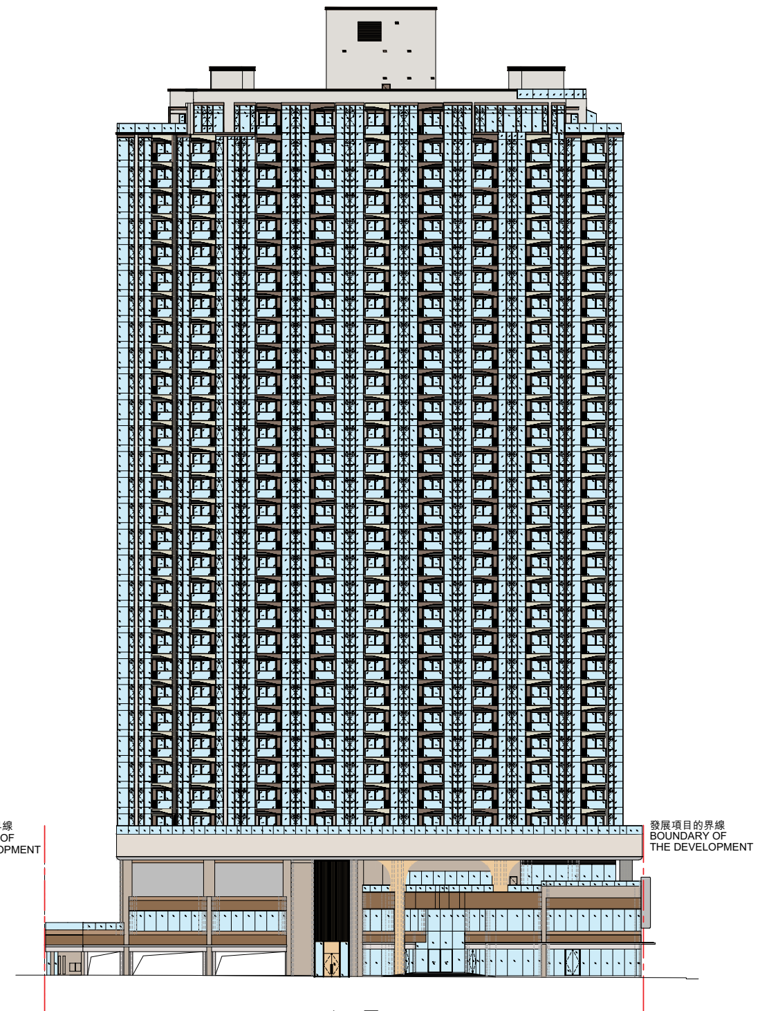
立面圖 D ELEVATION PLAN D
