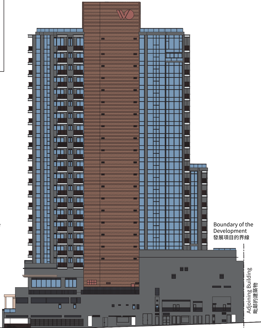
Elevation C C 立面圖
