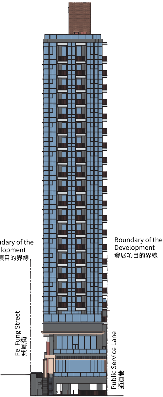
Elevation B B 立面圖
