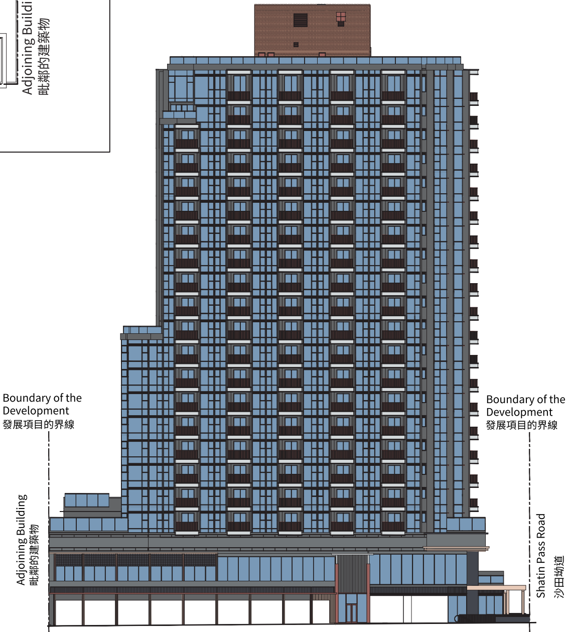
Elevation A A 立面圖
