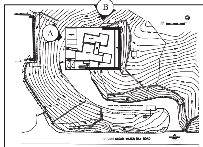
Key Plan 索引圖:
