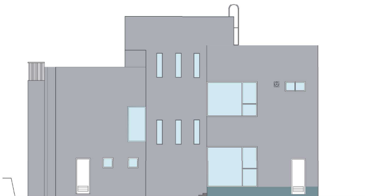
Elevation D 立面圖D
