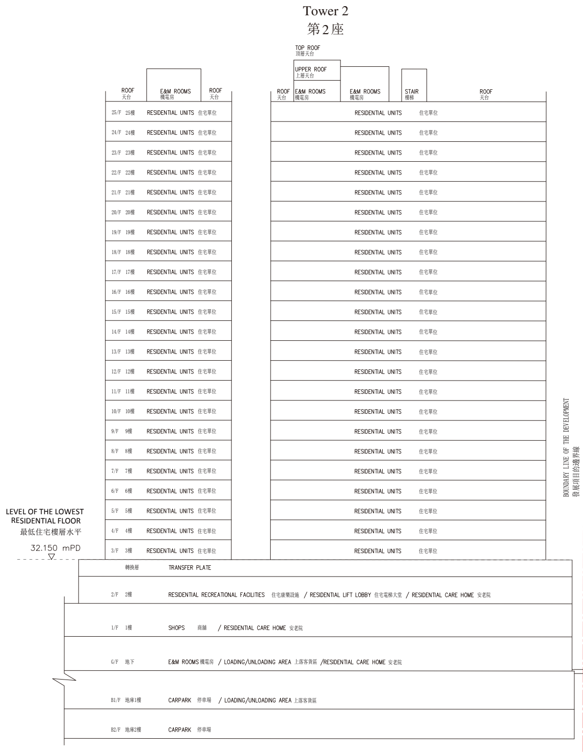
CROSS-SECTION PLAN 4 橫截面圖 4
