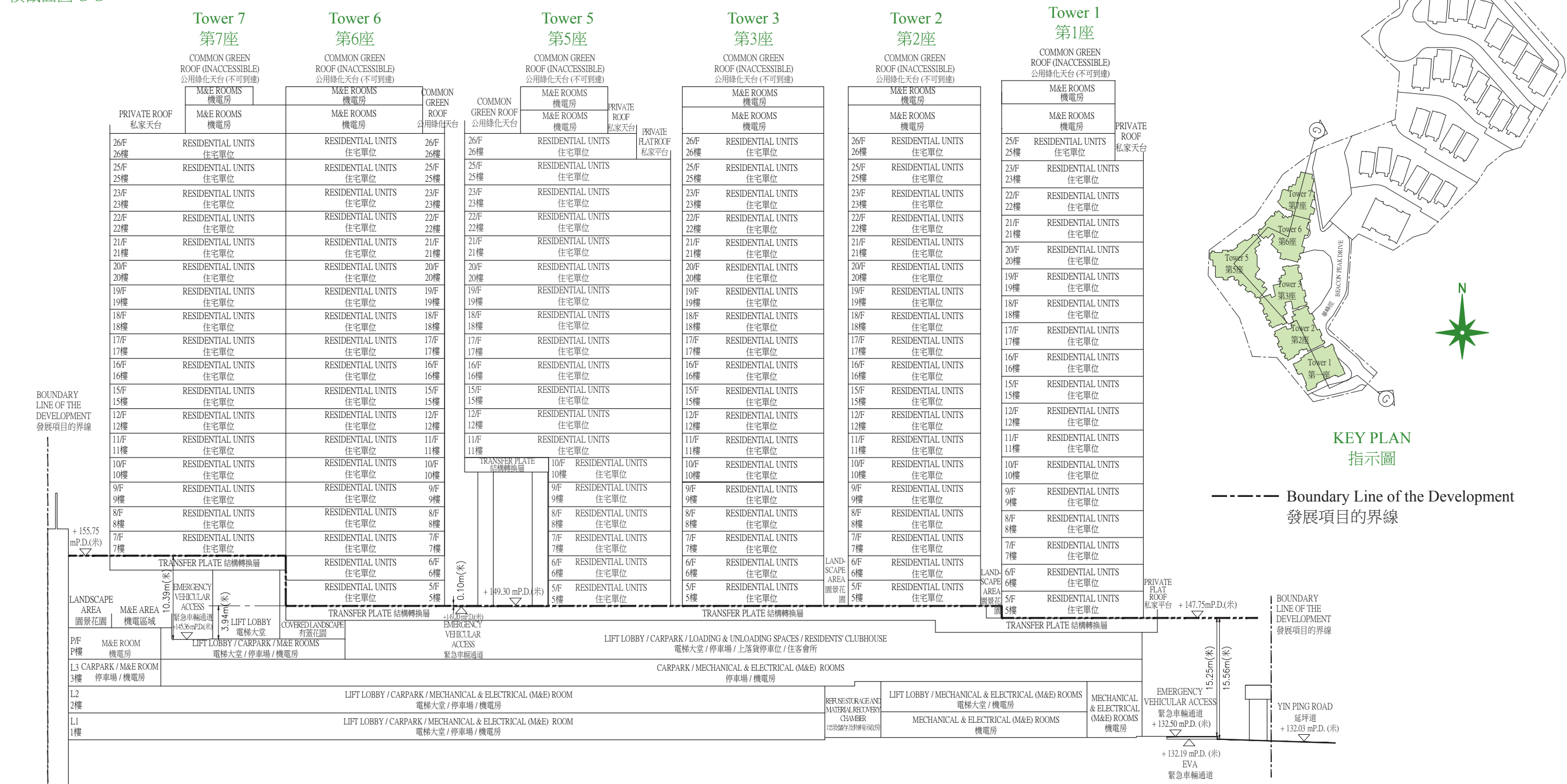
Cross-Section Plan G-G 橫截面圖 G-G
