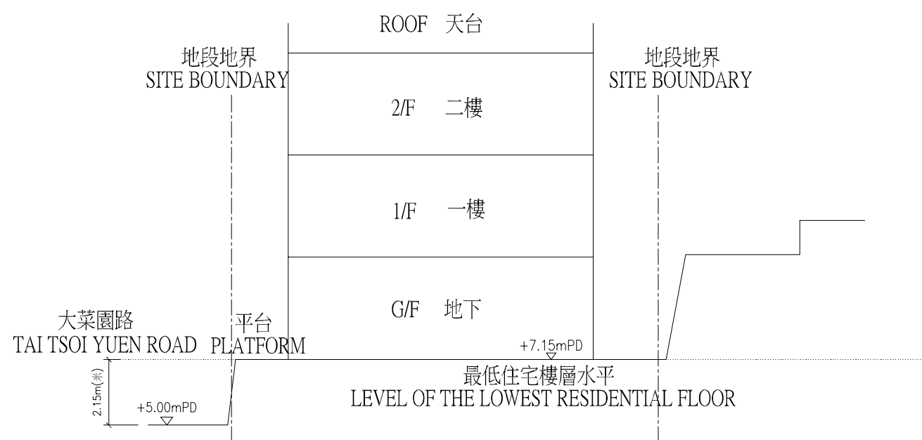
CROSS-SECTION PLAN E-E 橫截面圖 E-E
