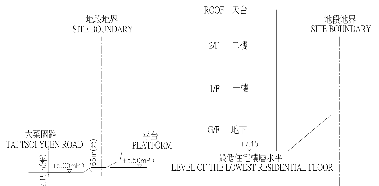
CROSS-SECTION PLAN A-A 橫截面圖 A-A
