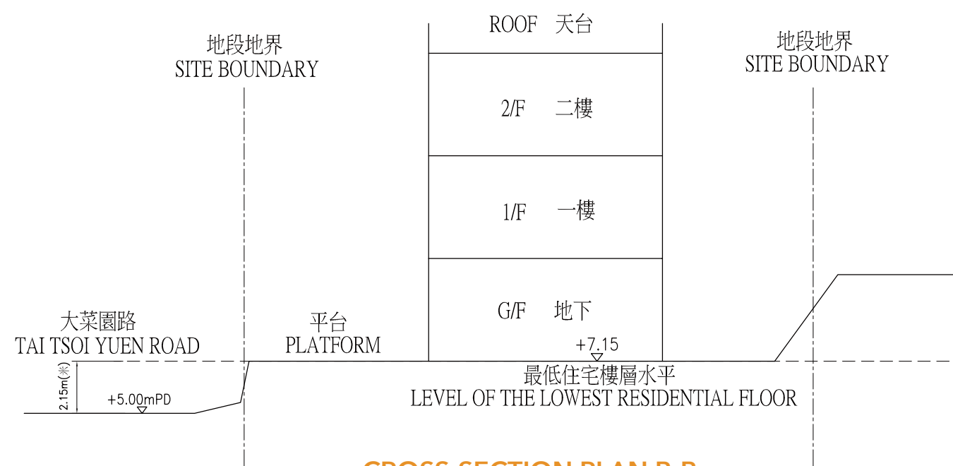
CROSS-SECTION PLAN B-B 橫截面圖 B-B
