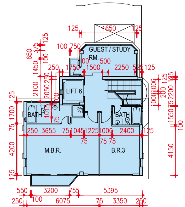
2/F PLAN 2樓平面圖
