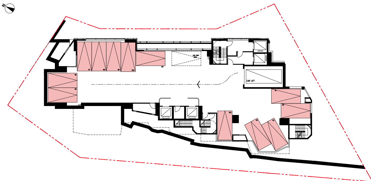
2樓平面圖 2/F Floor Plan
