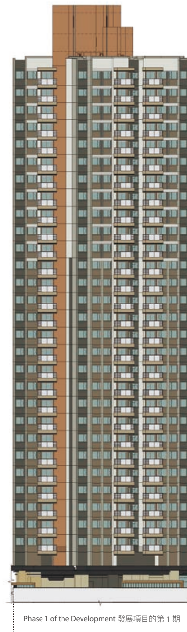
Elevation 2 立面圖 2
