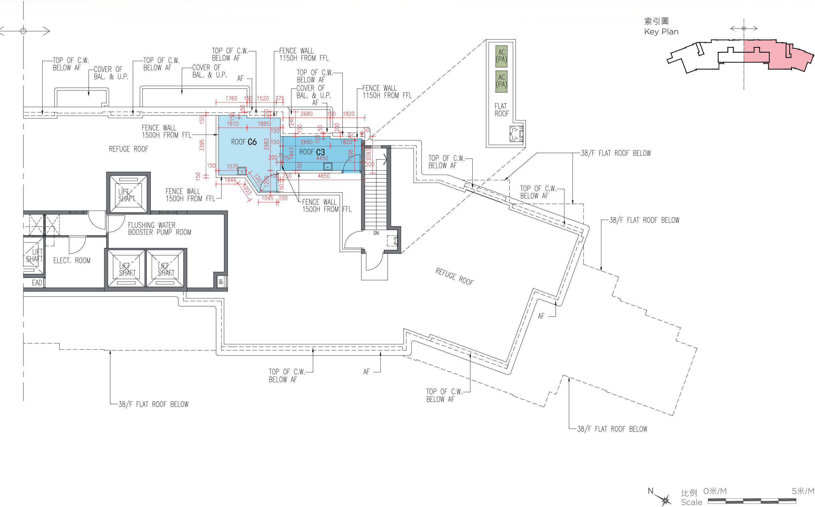
天台 平面圖 ROOF Plan
