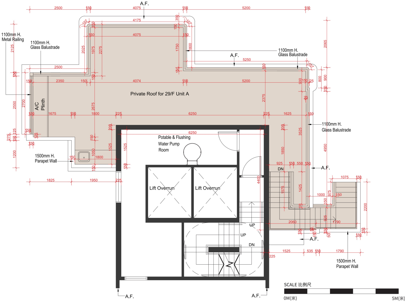
Roof Floor Plan 天台樓面平面圖
